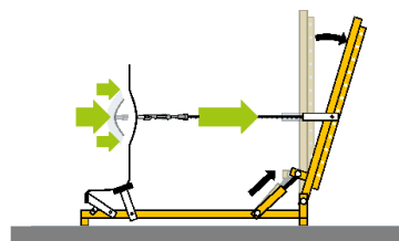
Système hydraulique de tirage
