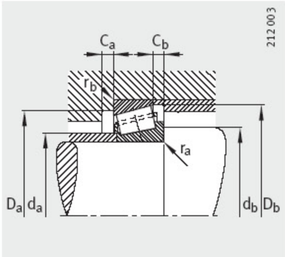
Cotes de montage
