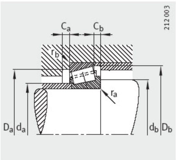
Cotes de montage
