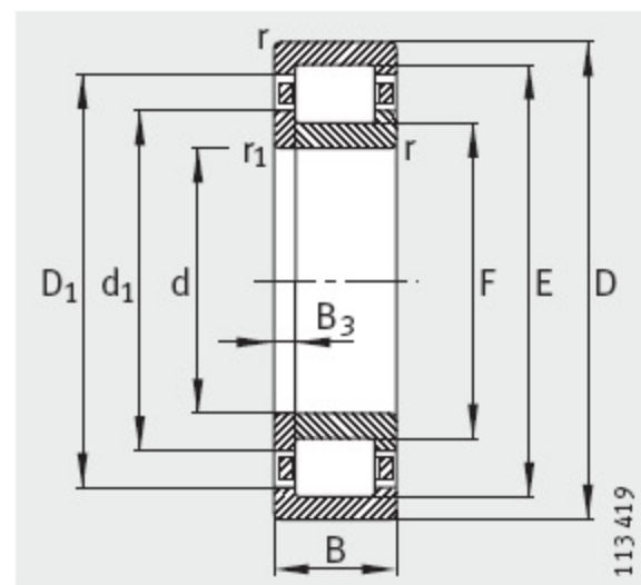
NUP Roulements pour paliers fixes
