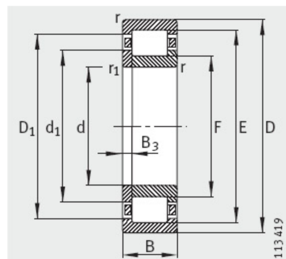
NUP Roulements pour paliers fixes
