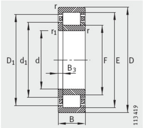
NUP Roulements pour paliers fixes
