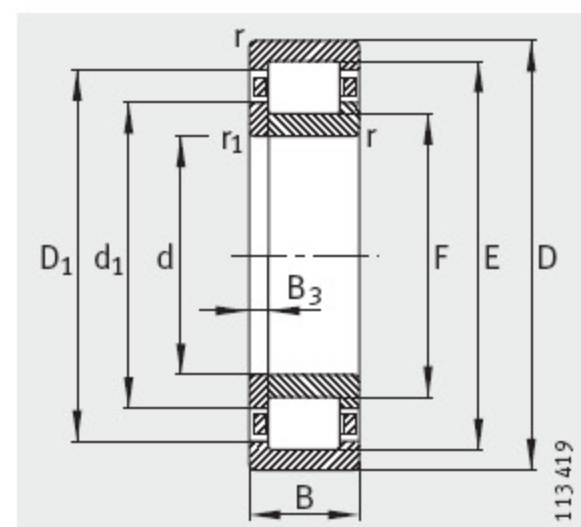
NUP Roulements pour paliers fixes
