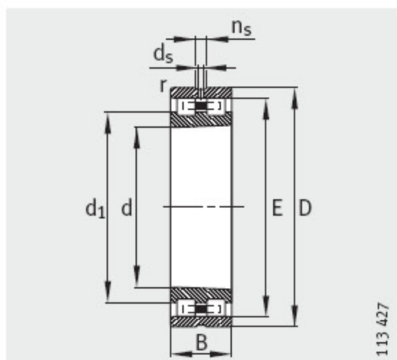
NN30..-AS-K-M-SP Cône 1:12
