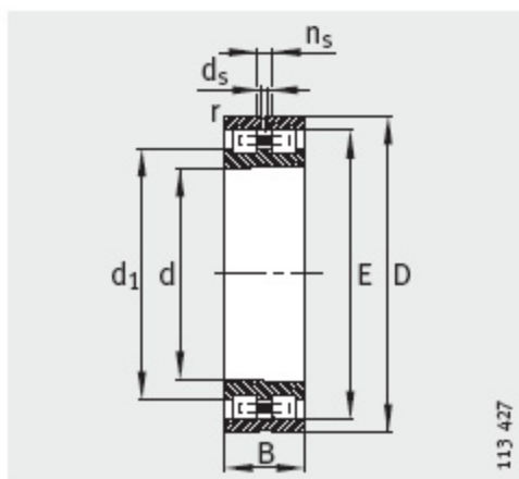
NN30..-AS-K-M-SP Cône 1:12
