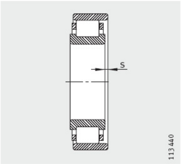
1) Déport axial «s» pour N et NU
