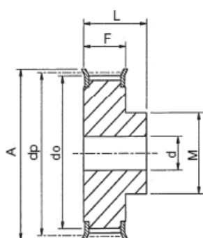
Type 1F (Steel)
